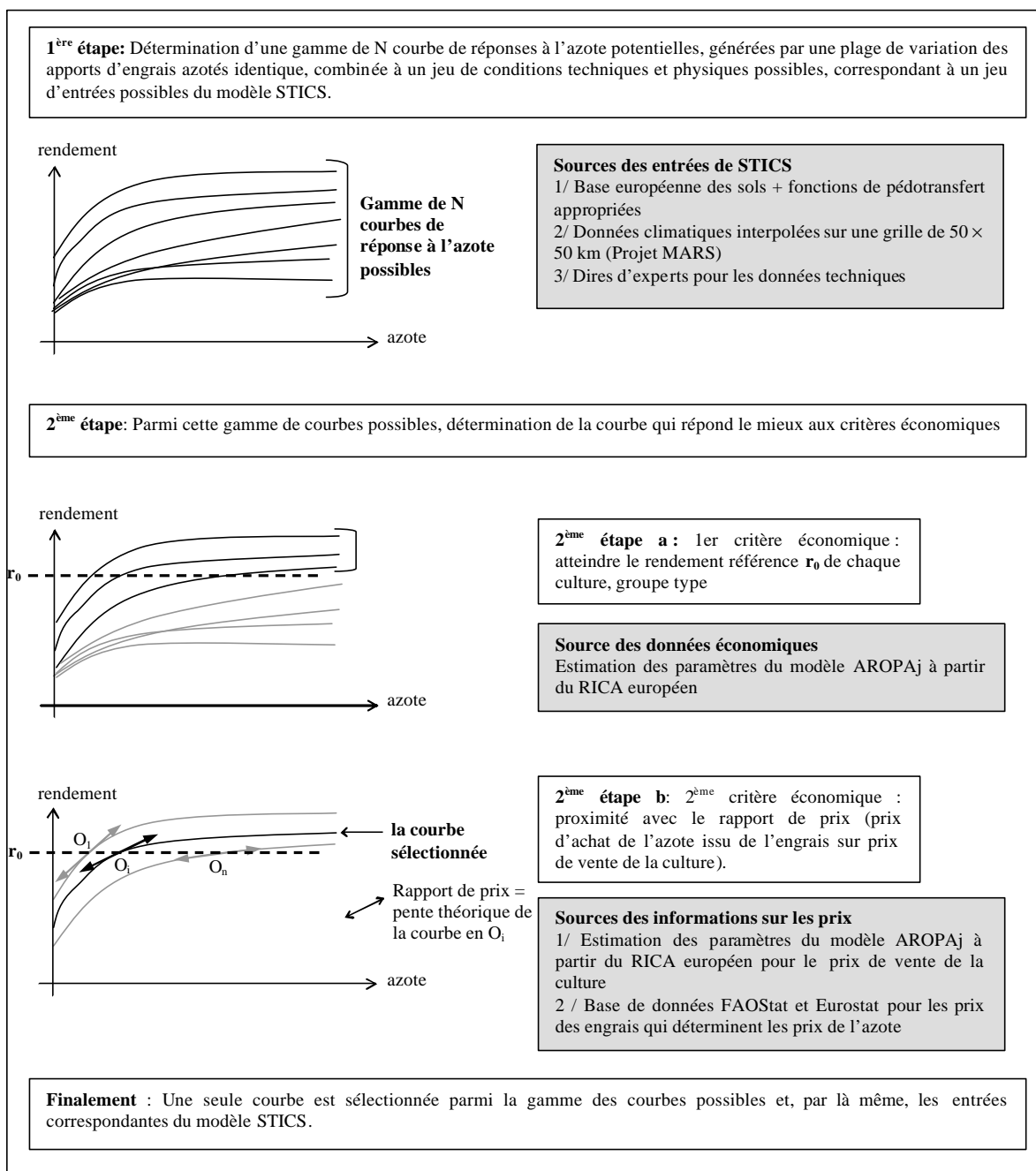
Figure 3.2 La méthode de construction de la courbe de réponse à l'azote pour une culture d'un groupe type, par la combinaison des modèles STICS et AROPAj.
