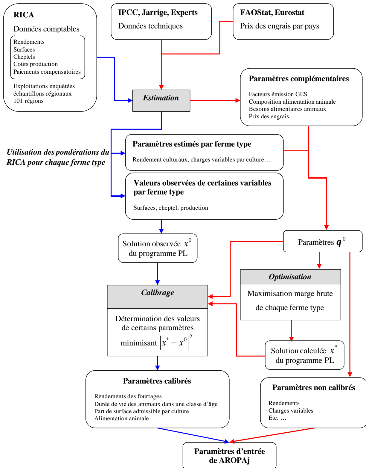
Figure 1.3 Elaboration des données utilisées par AROPAj
