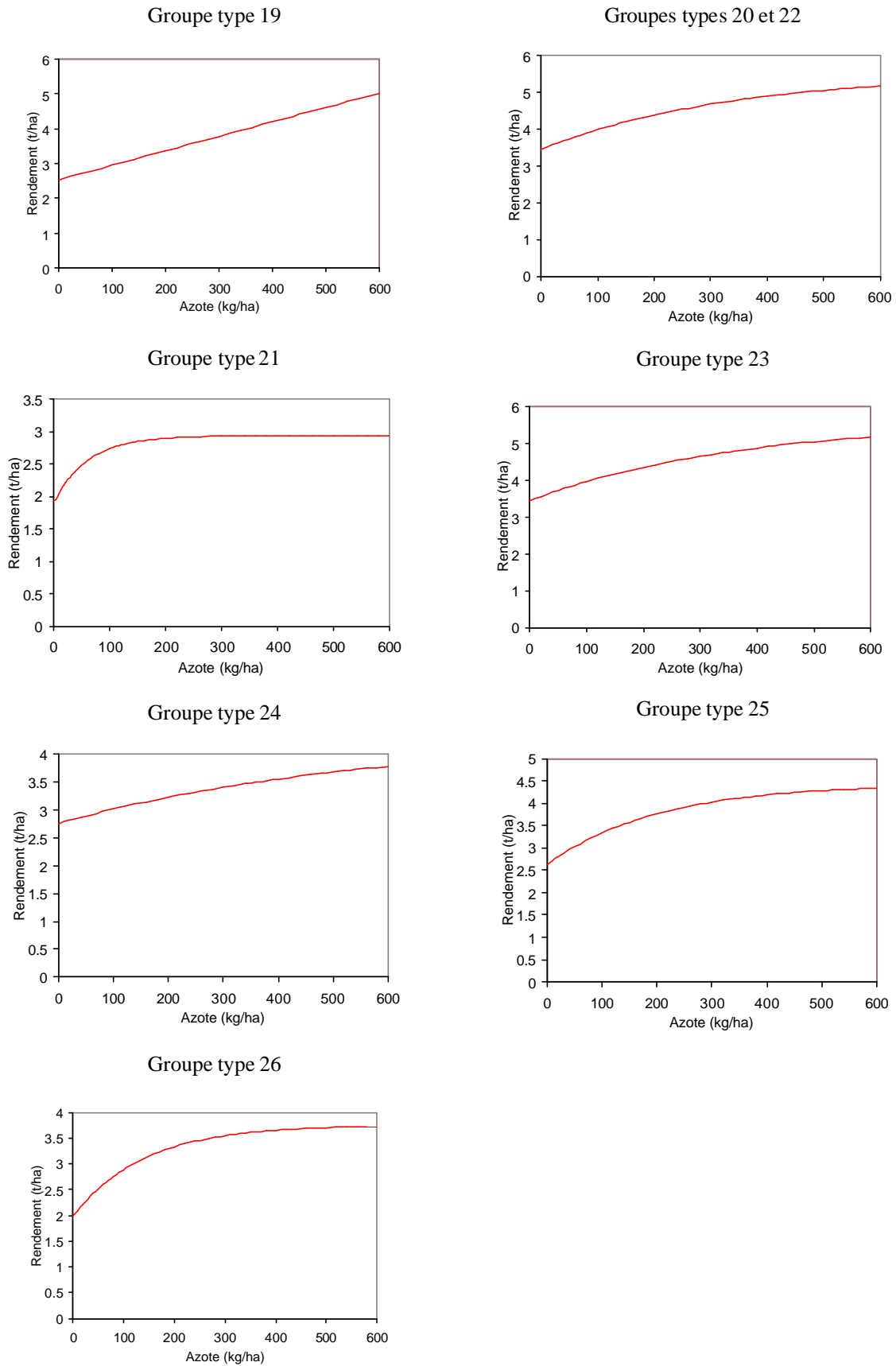
Figure 4.14 Les courbes de réponse à l'azote du blé tendre des groupes types "éleveurs" de Midi-Pyrénées
