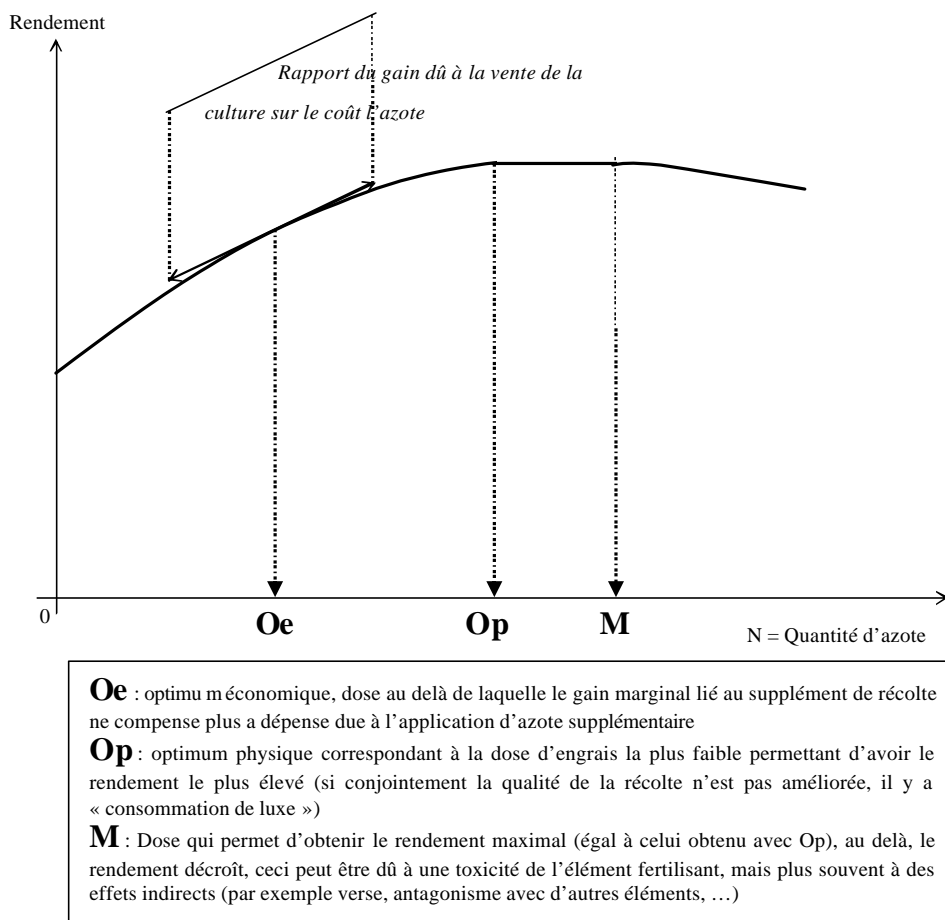
Figure 1.11 Courbe de réponse du rendement à l'azote attendue par l'agronome (d'après l'Encyclopédie des techniques agricoles, 1999)
