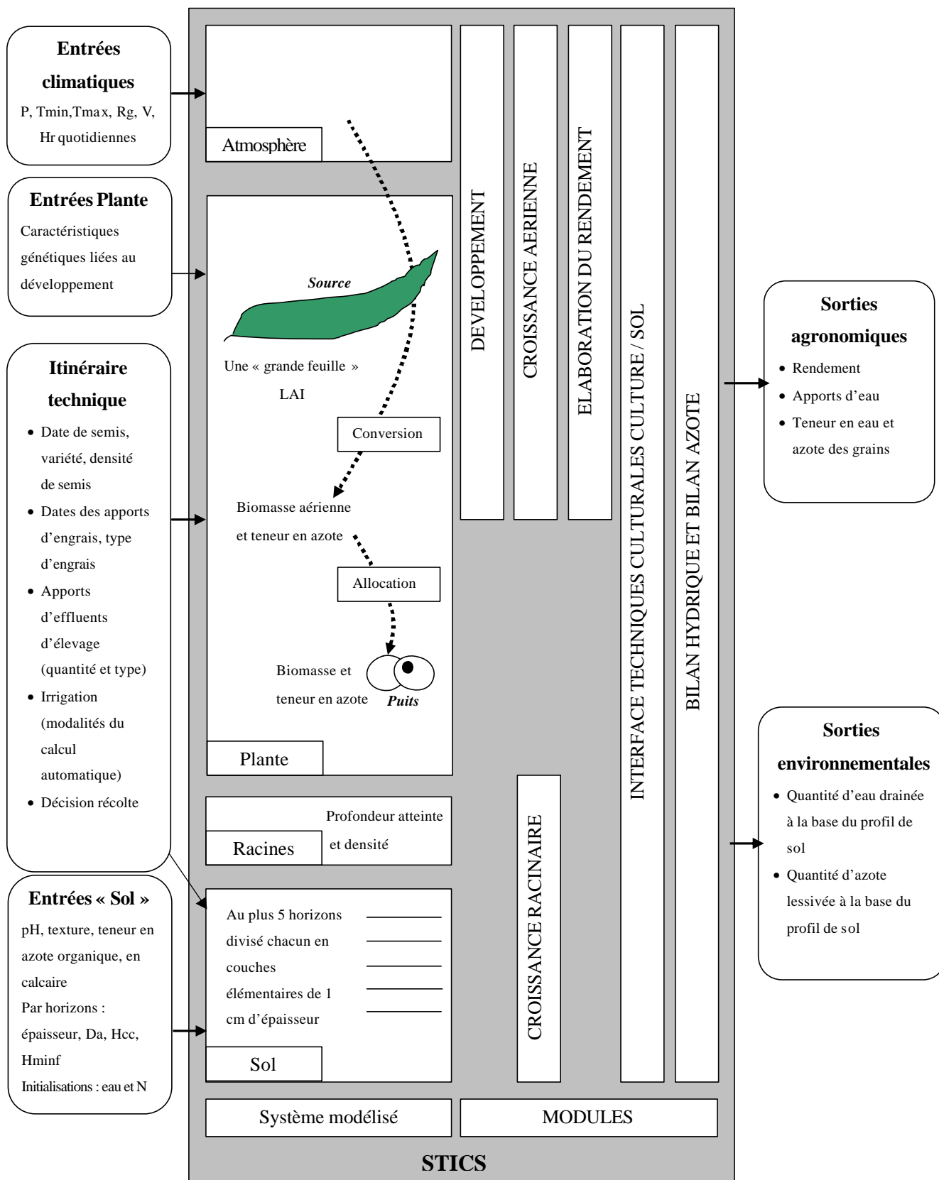
Figure 1.5 Fonctionnement général de STICS : les entrées, le système modélisé, les modules et les sorties
